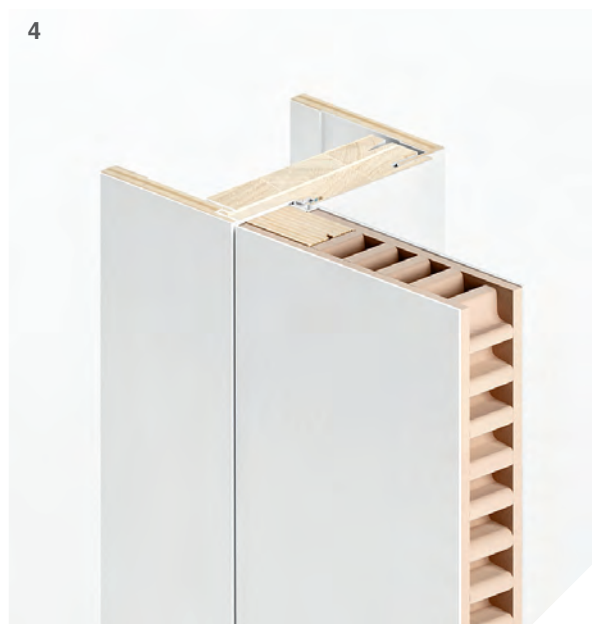
3 Spaccato porta Trend S registrazione lato interno Trend S door section adjusting internal side
